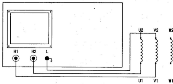
图 3-1 \Phi (相) 接法
