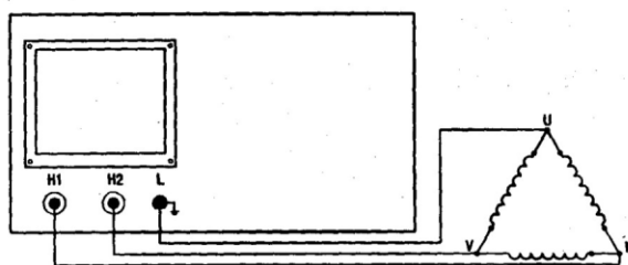
图 3-3 Δ（角）接法
