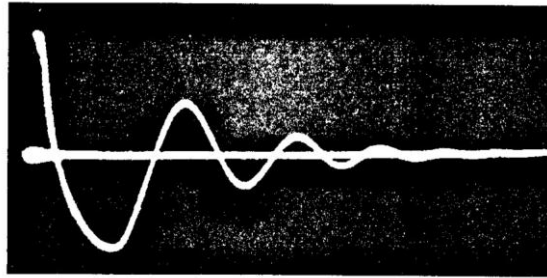
图 3-7 短路波形
